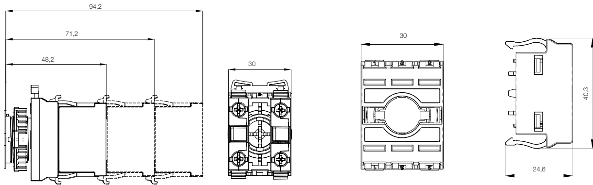
AF3F + 1..3x Blocos de contatos BC_F
