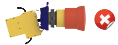
Bloco NÃO montado corretamente na flange.
