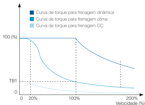
Gráfico típico de torque de frenagem x rotação para um motor de 10 cv / 7,5 kW acionado por um CFW11
