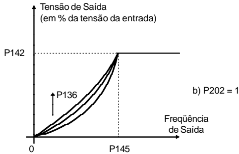
Figura 6.6 a) b) - Curva V/F e detalhe do boost de torque manual (compensação IxR)
