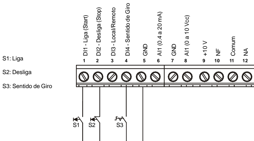
Figura 3.11 – Conexão do Controle para Acionamento 3
