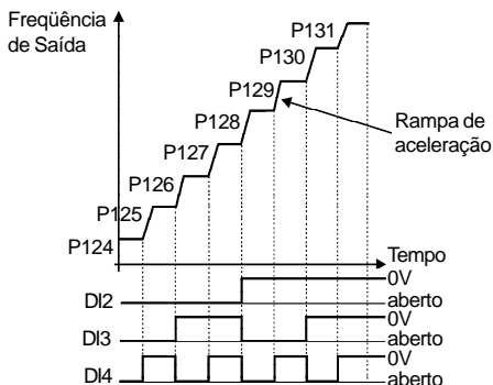
Figura 6.5 - Diagrama de tempo da função multispeed
