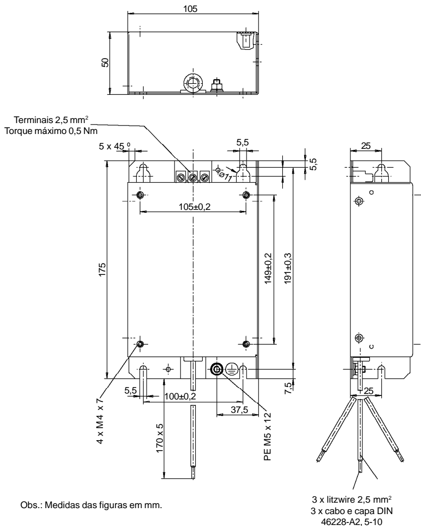
Figura 3.14 a) - Desenhos dos filtros footprint / booksize
