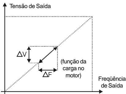
Figura 6.10 - Curva V/F com compensação de escorregamento
