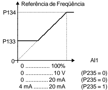
Figura 6.17 a) - Determinação da referência de frequência a partir da entrada analógica AI1
