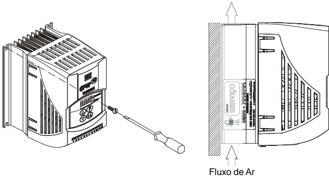
Figura 3.3 - Procedimento de instalação do CFW-10
