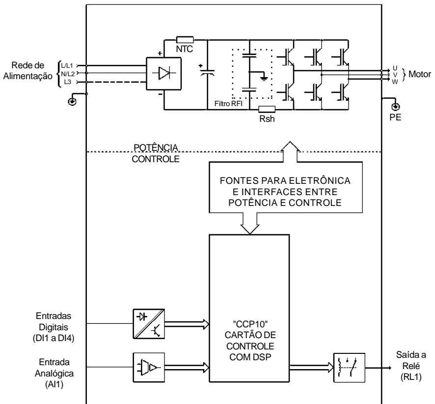
Figura 2.1 - Diagrama de Blocos do CFW-10 modelos 1,6 A, 2,6 A e 4,0 A / 200-240 V (monofásico) e 1,6 A, 2,6 A, 4,0 A e 7,3 A / 200-240 V (trifásico)
