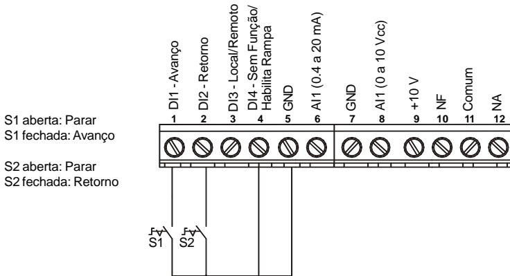
Figura 3.12 – Conexão do Controle para Acionamento 4
