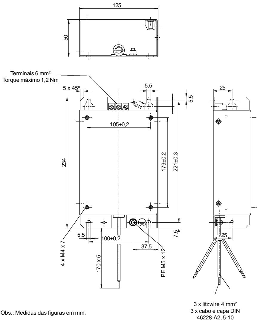
Figura 3.14 c) - Desenhos dos filtros footprint / booksize
