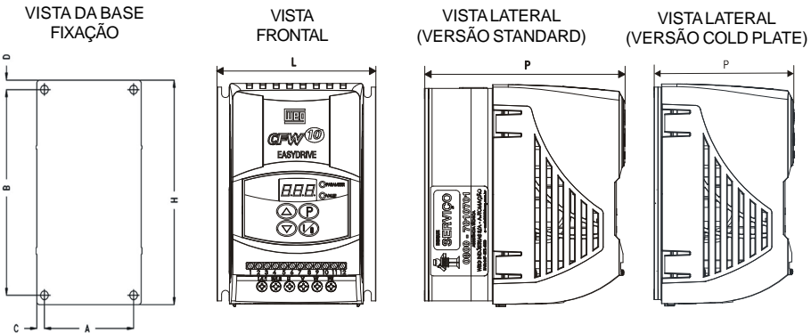
Figura 3.1 - Dimensional do CFW-10 - Mecânicas 1, 2 e 3
