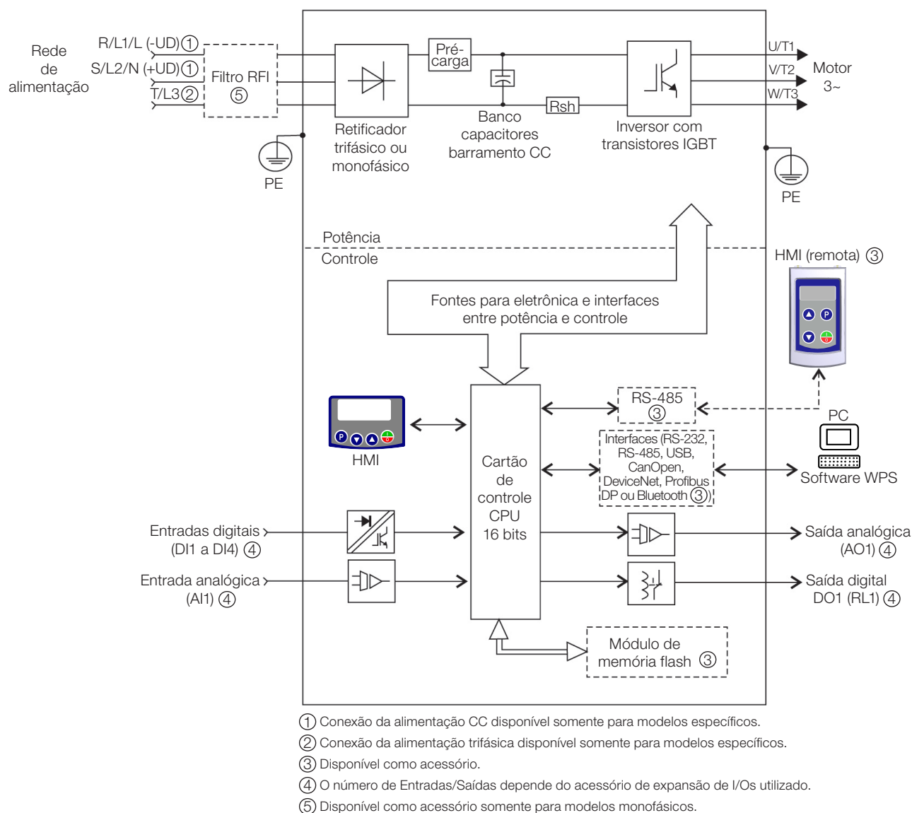
Figura 3.1: Blocodograma do CFW300 para mecânica A 220 V
