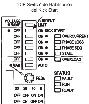
Figura 4.2 - Habilitación del Kick Start
