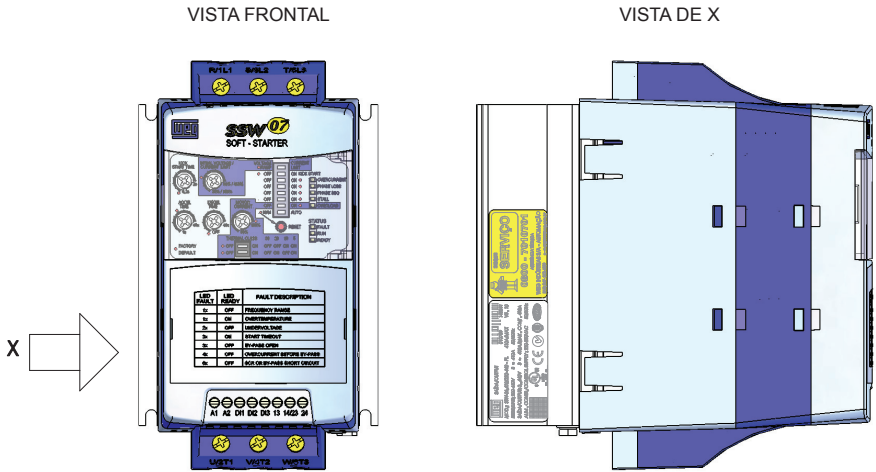
Figura 2.4 - Ubicación de las etiquetas
