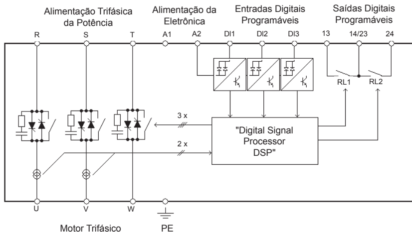
Figura 2.2 - Bloco diagrama da Soft-Starter SSW-07
