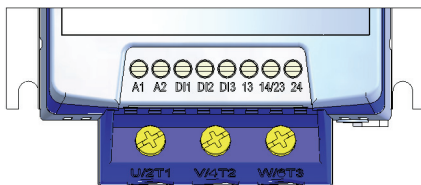
Figura 3.9 - Bornes de controle da SSW-07
