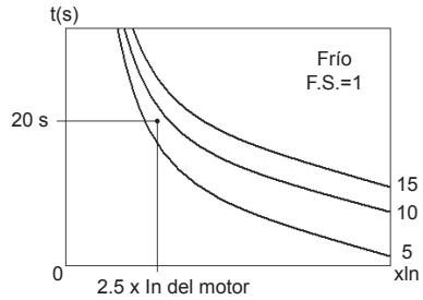
Figura 5.6 - Verificando la clase mínima en las curvas a frío
