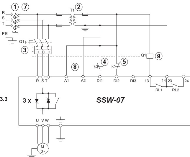
Figura 3.11 - Acionamento sugestivo com comandos por entradas digitais a três fios e disjuntor de isolamento da potência
