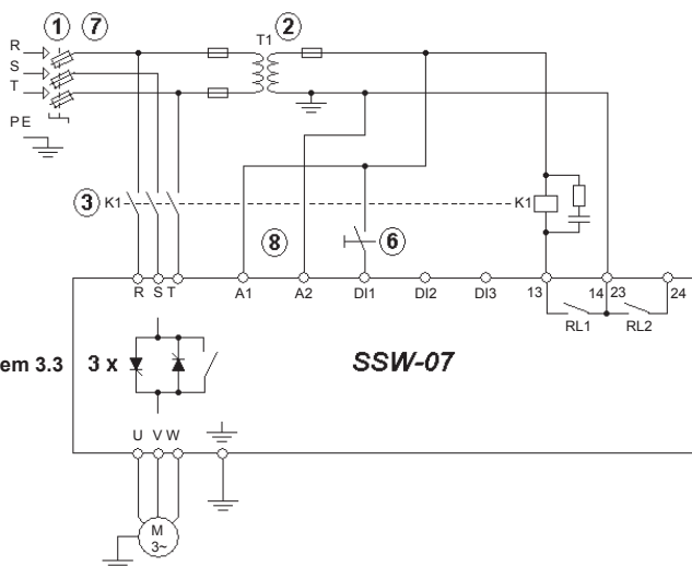
Figura 3.10 - Acionamento sugestivo com comandos por entradas digitais a dois fios e contator de isolamento da potência
