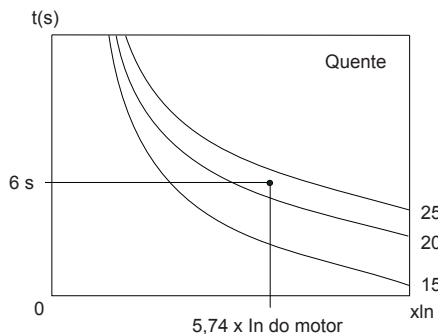
Figura 5.8 - Verificando a máxima classe térmica a quente, considerando o F.S.
