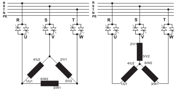
Figura 3.7 - Soft-Starter SSW-07 com ligação padrão
