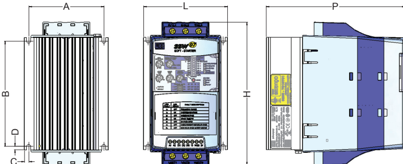
Figura 3.1 - Dimensional da SSW-07
