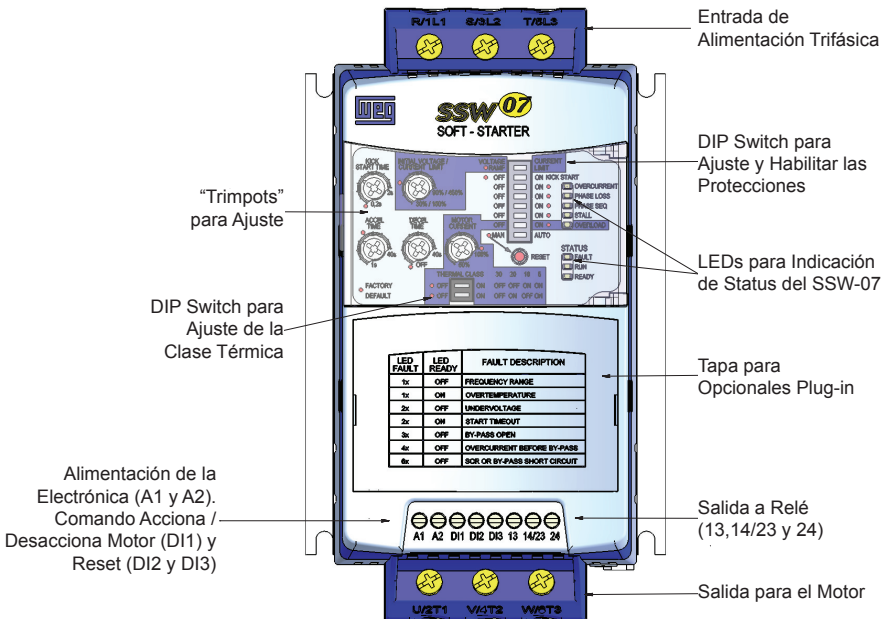
Figura 2.1 - Vista frontal del SSW-07
