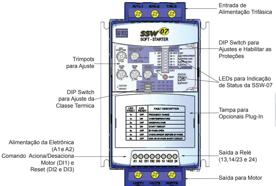
Figura 2.1 - Vista frontal da SSW-07
