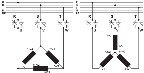
Figura 3.7 - Arrancador Suave SSW-07 con conexión padrón
