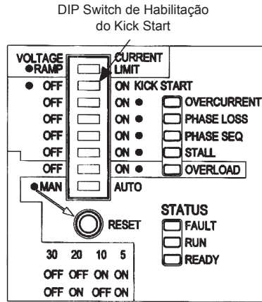
Figura 4.2 - Habilitação do Kick Start
