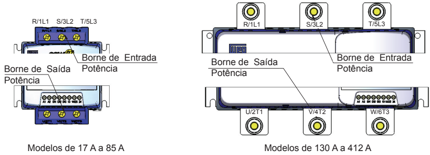
Figura 3.5 - Bornes de potência
