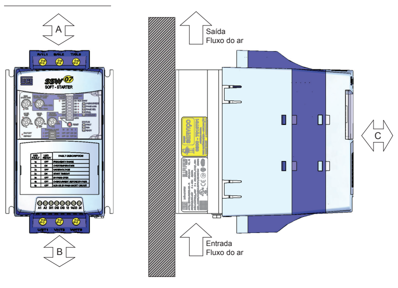
Figura 3.2 - Espaços livres para ventilação
