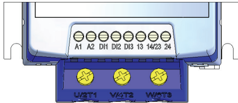
Figura 3.9 - Terminales de control de la SSW-07
