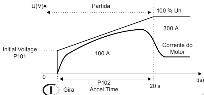
Figura 5.5 - Curva típica de corrente numa partida por rampa de tensão
