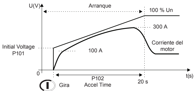
Figura 5.5 - Curva típica de corriente en un arranque por rampa de tensión
