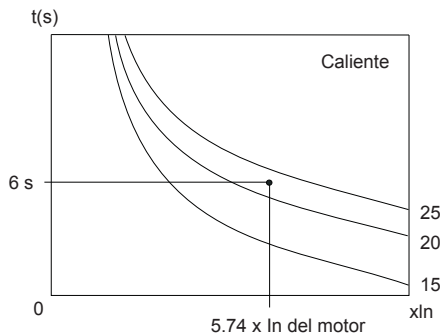
Figura 5.8 - Verificando la máxima clase térmica a caliente, considerando el factor de servicio
