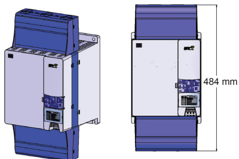
Figura 7.2 - Kit IP20 mecánica 4
