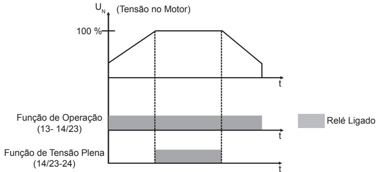
Figura 4.11 - Funcionamento das saídas a relé
