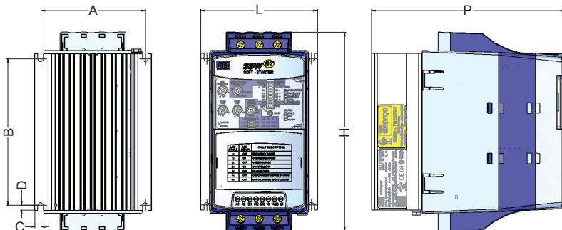
Figura 3.1 - Dimensional de la SSW-07
