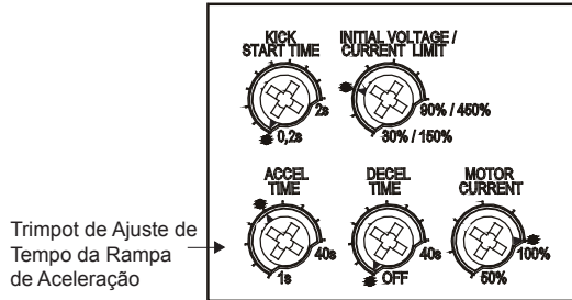
Figura 4.5 - Ajuste do tempo da rampa de aceleração
