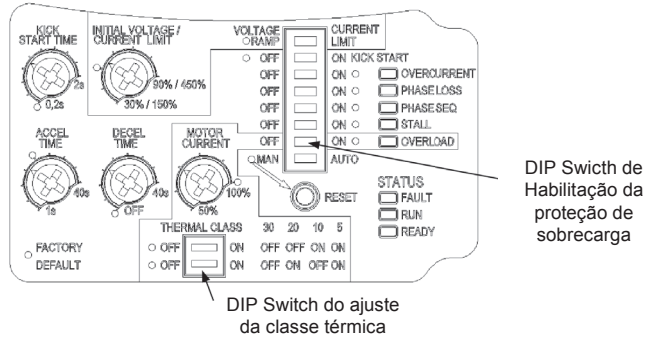
Figura 4.10 - Habilitação e ajuste de proteção de sobrecarga
