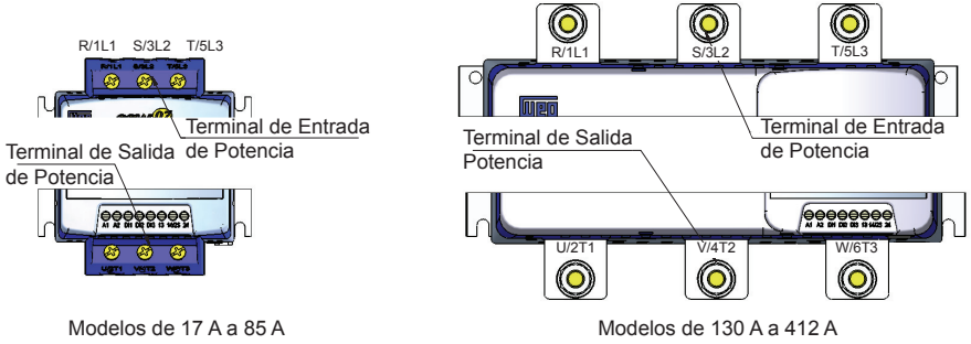
Figura 3.5 - Terminales de potencia
