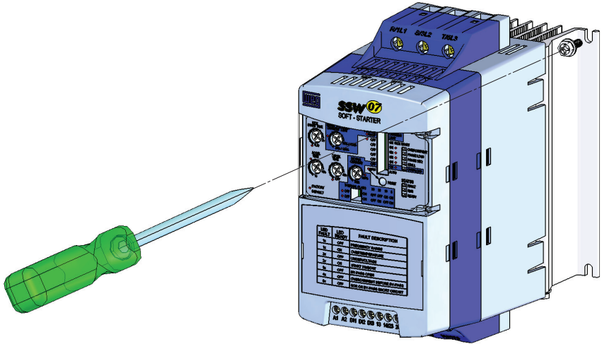
Figura 3.3 - Procedimento de instalação da SSW-07 em superfície
