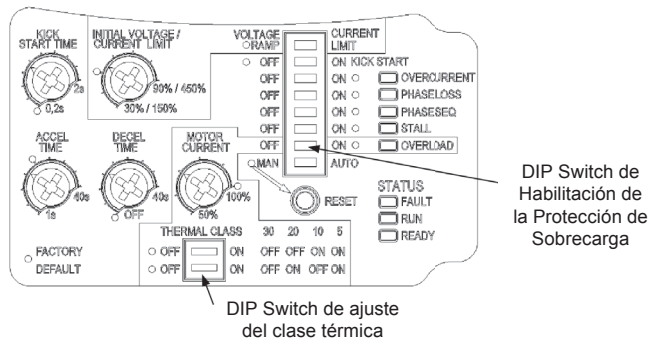
Figura 4.10 - Habilitación e ajuste del protección de sobrecarga
