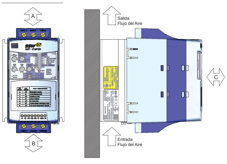
Figura 3.2 - Espacios libres para la ventilación
