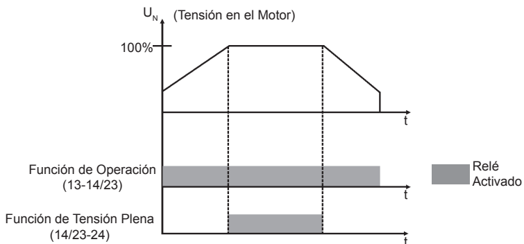
Figura 4.11 - Funcionamiento de las salidas a relé
