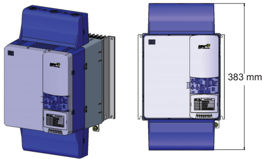
Figura 7.1 - Kit IP20 mecânica 3
