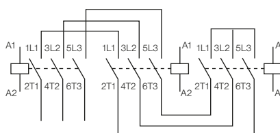
Diagrama elétrico
