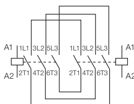
Diagrama elétrico
