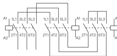
Diagrama elétrico
